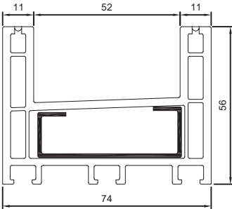
Marco corredera 2 hojas 7401
