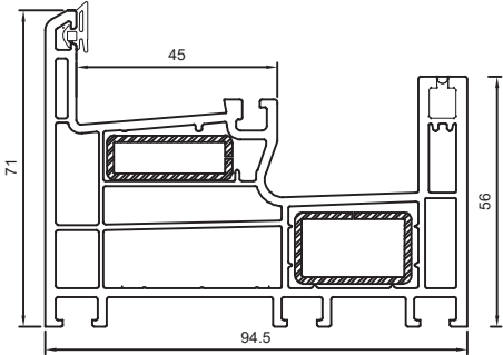
Marco monorriel 7411
