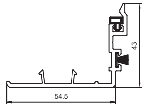
Traslapo hoja corredera chica 7419
