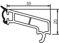
Junquillo para vidrio 4mm 6306
